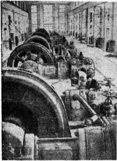
Тульская область. Молодой гигант советской индустрии — Щекнинский химический комбинат, раскинувшийся под Тулой, быстро набирает силы. Здесь сдан в эксплуатацию комплекс цехов по производству аммиака. На снимке: аммиачные компрессоры цеха производства мочевины. Фото П. Маслова. Фотохроника ТАСС
