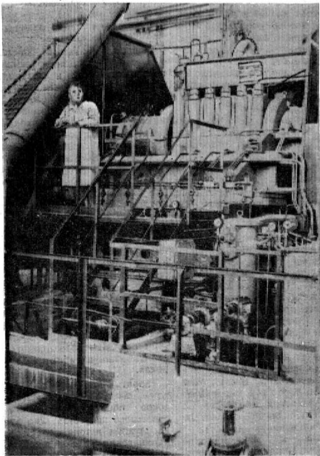
ПОСЕЛОК КОВДОР. Шековая дробилка отделения крупного дробления обогатительной фабрики.
